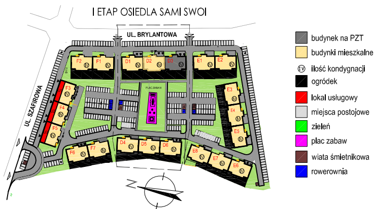
PROJEKT ZAGOSPODAROWANIA TERENU
