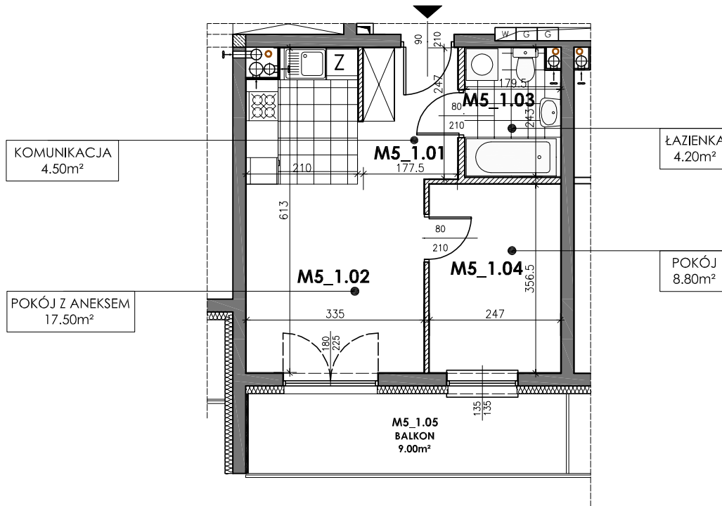
RZUT LOKALU
