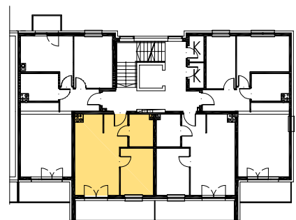
RZUT KONDYGNACJI
