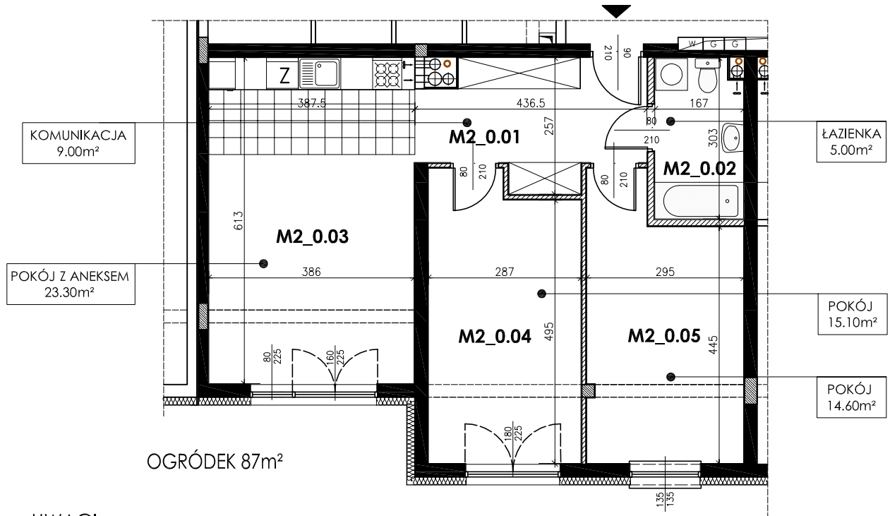
RZUT LOKALU
