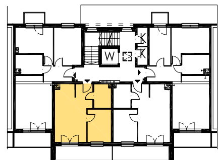
RZUT KONDYGNACJI
