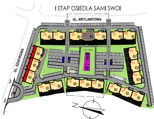
PROJEKT ZAGOSPODAROWANIA TERENU
