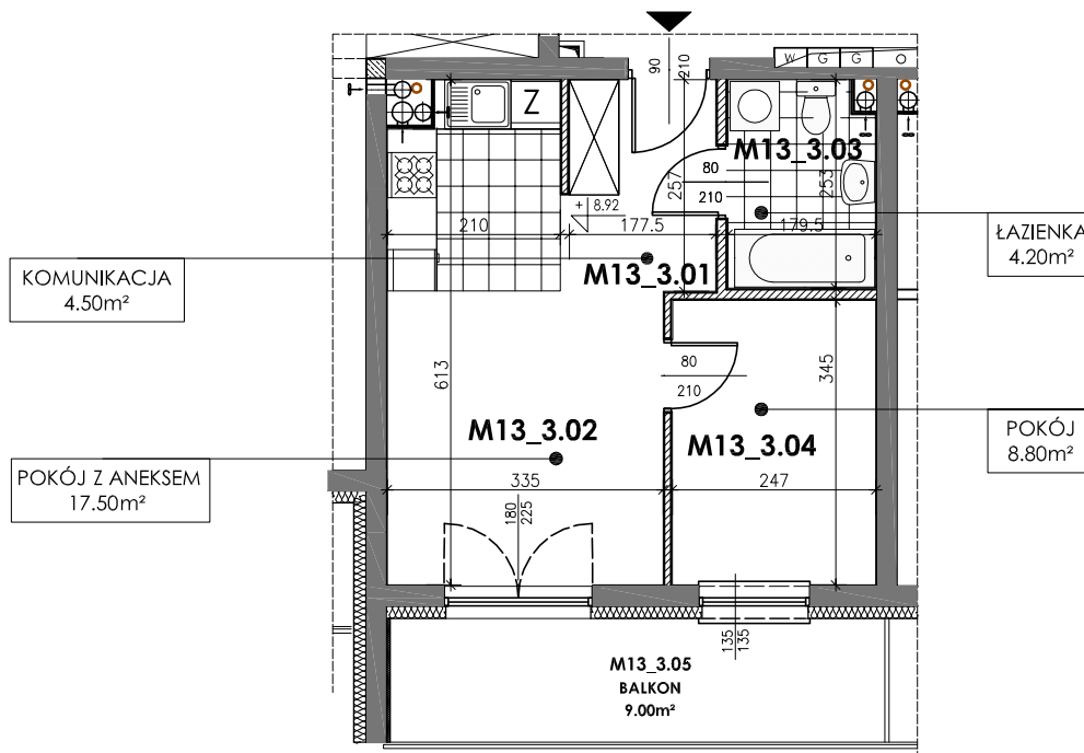
RZUT LOKALU
