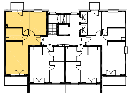
RZUT KONDYGNACJI
