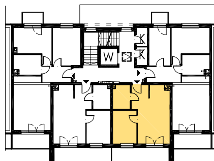
RZUT KONDYGNACJI
